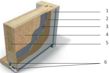
BRANNDØR (62mm) TREND TETT SLETT EI30/35DB 1. Malt ytterside 2. HDF plate 3. Alu fuktsperre 4. Brannhemmende plate 5. Rockwool 6. Alu/tre terskel
