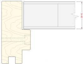
Profil av kompakt dør
