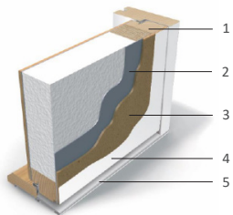
STANDARD (62mm) 1. Ramtre i furu og lamellimt finér 2. Polystyren 3. Aluminium 4. HDF-plate (High Density Fibreboard) 5. Toppstrøk
