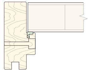
Profil av kompakt dør
