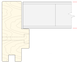
Profil av kompakt dør
