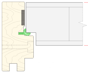
Karmprofil av B60/Rw38dB dør
