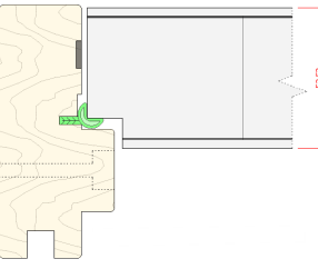
Karmprofil av klimadør. B30/Rw38dB dør, 52mm dørblad
