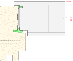
Karmprofil av B30/Rw43dB dør
