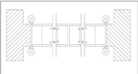
Profil av tofløyet pendeldør
