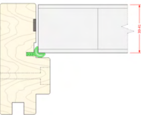
Karmprofil av B30/Rw38dB dør 40mm dørblad
