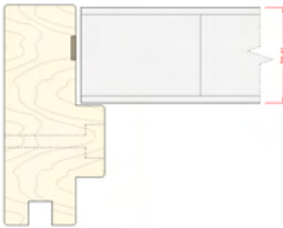
Karmprofil av B30 dør
