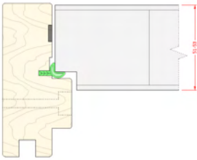
Karmprofil av B30/Rw38dB dør 52mm dørblad
