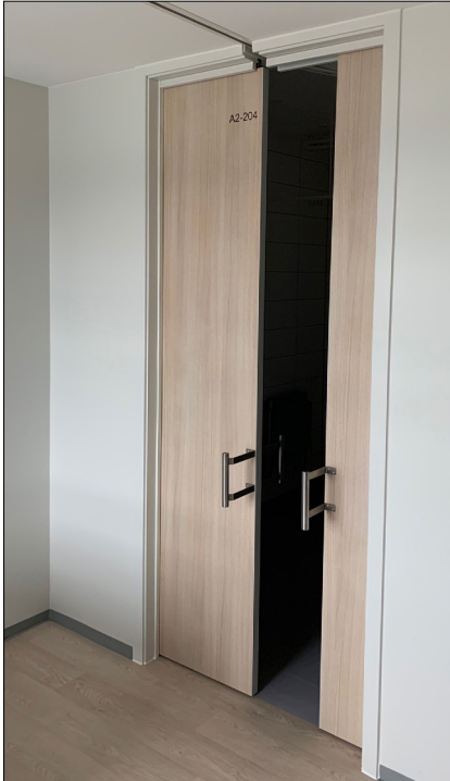
Sykehjem: 2-fløyet skyvedør til bad m/uttak i karm for takheis
