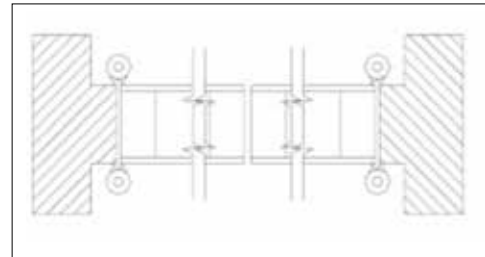
Profil av tofløyet pendeldør
